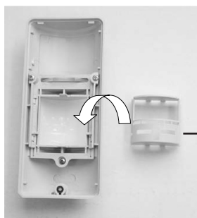
Filtro de imunidade para animais de estimação e tampa
