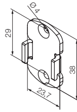
523.30002 Adattatore universale bianco compatibile con supporti Rollease della serie Skyline (interasse 29 mm).
