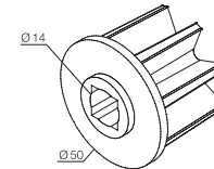
575.12150 Calotta senza perno per rullo Ø 50 mm.
