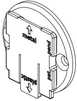
523.30000 Adattatore universale bianco per supporti Coulisse (interasse 29 mm).
