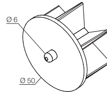
575.12050 Calotta con perno per rullo Ø 50 mm.
