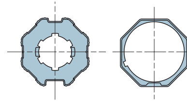
515.05200 Ottagonale 52x0,8 ruota + corona
