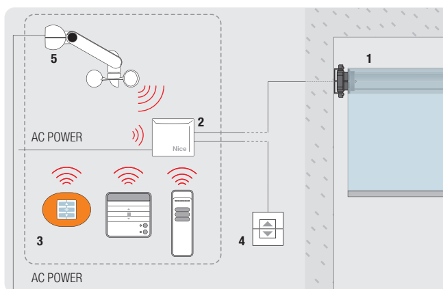
1. MOTORE TUBOLARE 2. CENTRALE SERIE MINDY TT4 3. TRASMETTITORE 4. PULSANTE "SALI/SCENDI" COLLEGATO ALLA CENTRALE SERIE MINDY TT4 5. ANEMOMETRO RADIO SERIE NEMO
