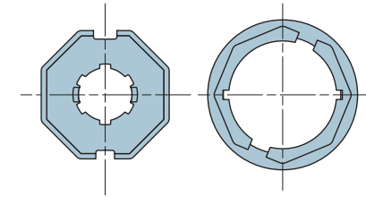
515.05700 Ottagonale 57x0,8 ruota + corona
