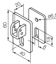
525.10087 max 30 Nm Kit supporto con staffa e sella per perno quadro 10 mm.
