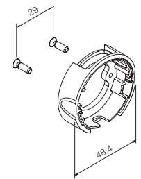
533.10010 Supporto compatto (nero).
